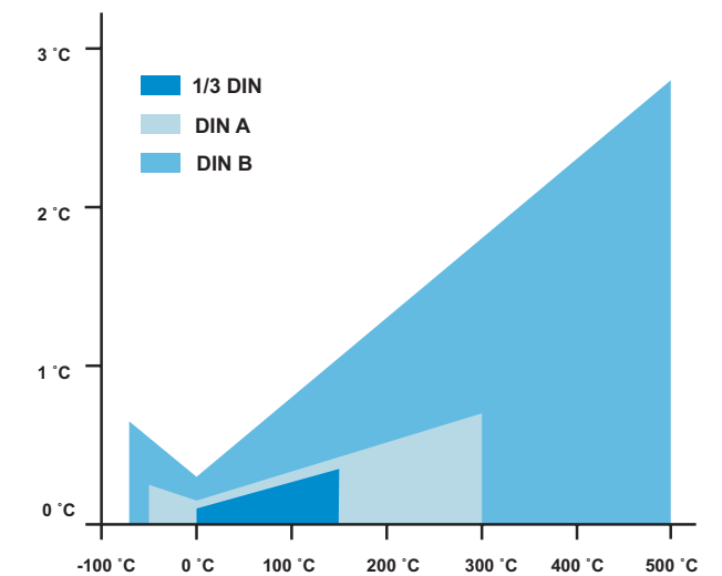
Классы точности платиновых тонкопленочных датчиков температуры, установленные DIN EN 60751
