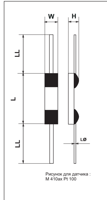
Точка измерения определена на расстоянии 8 мм от кромки тела датчика
