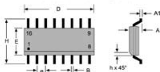
HMC1022—16-Pin SOIC
